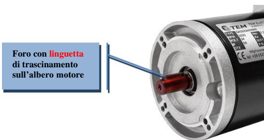
Fig. 3 : Albero motore
